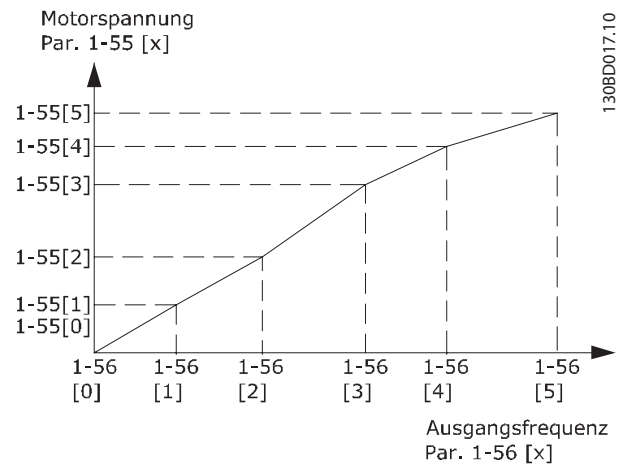
Abbildung 4.3 U/f-Kennlinien
